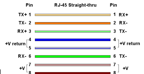
Pin-Belegung Kat. 5 Netzwerkkabel
