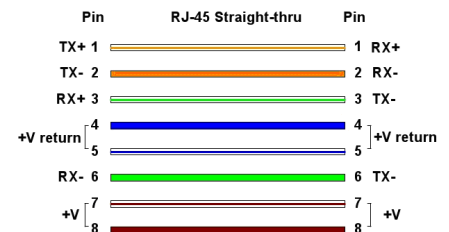
pedinatura cavo di rete CAT 5
